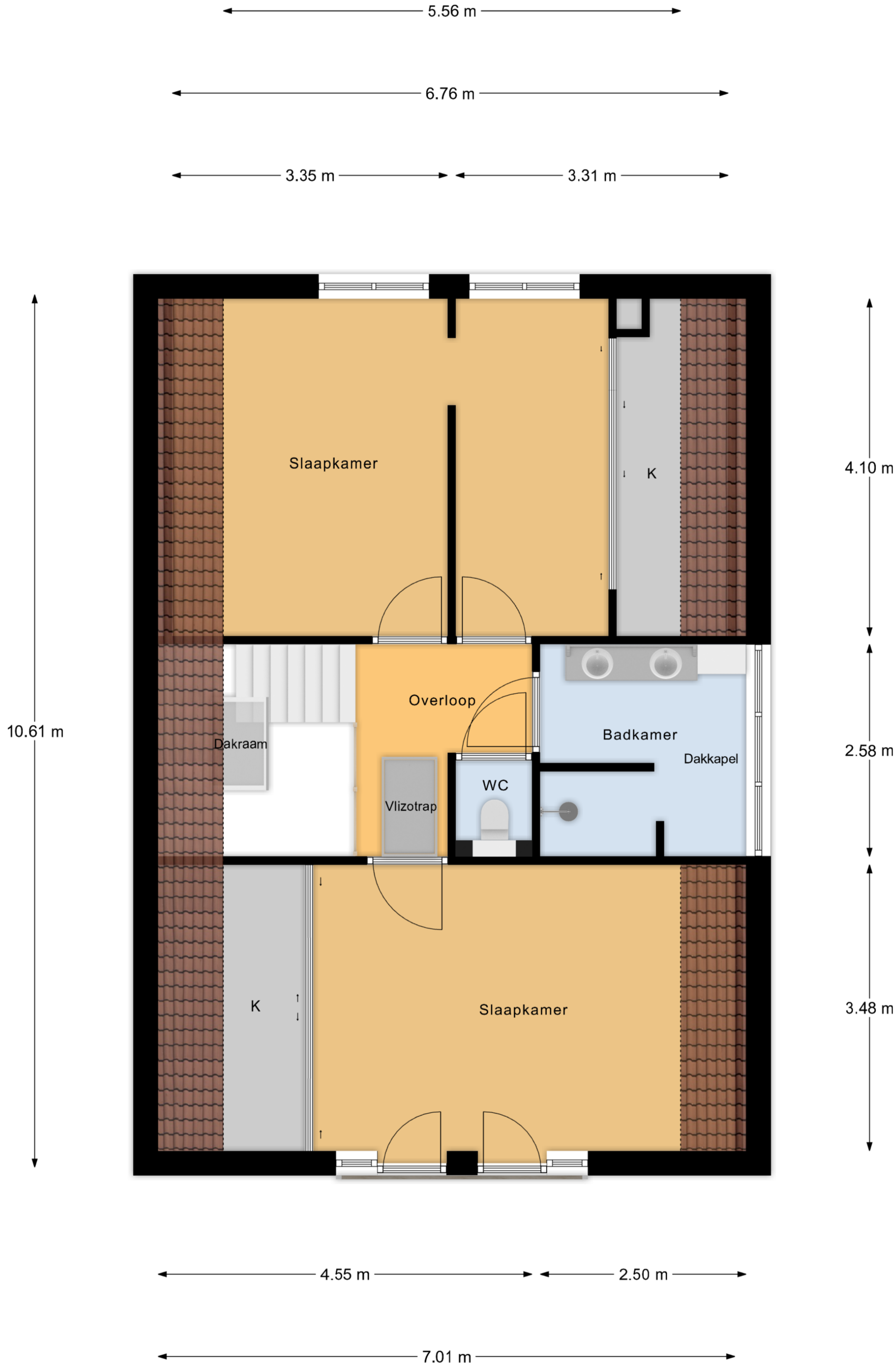
1e Verdieping
