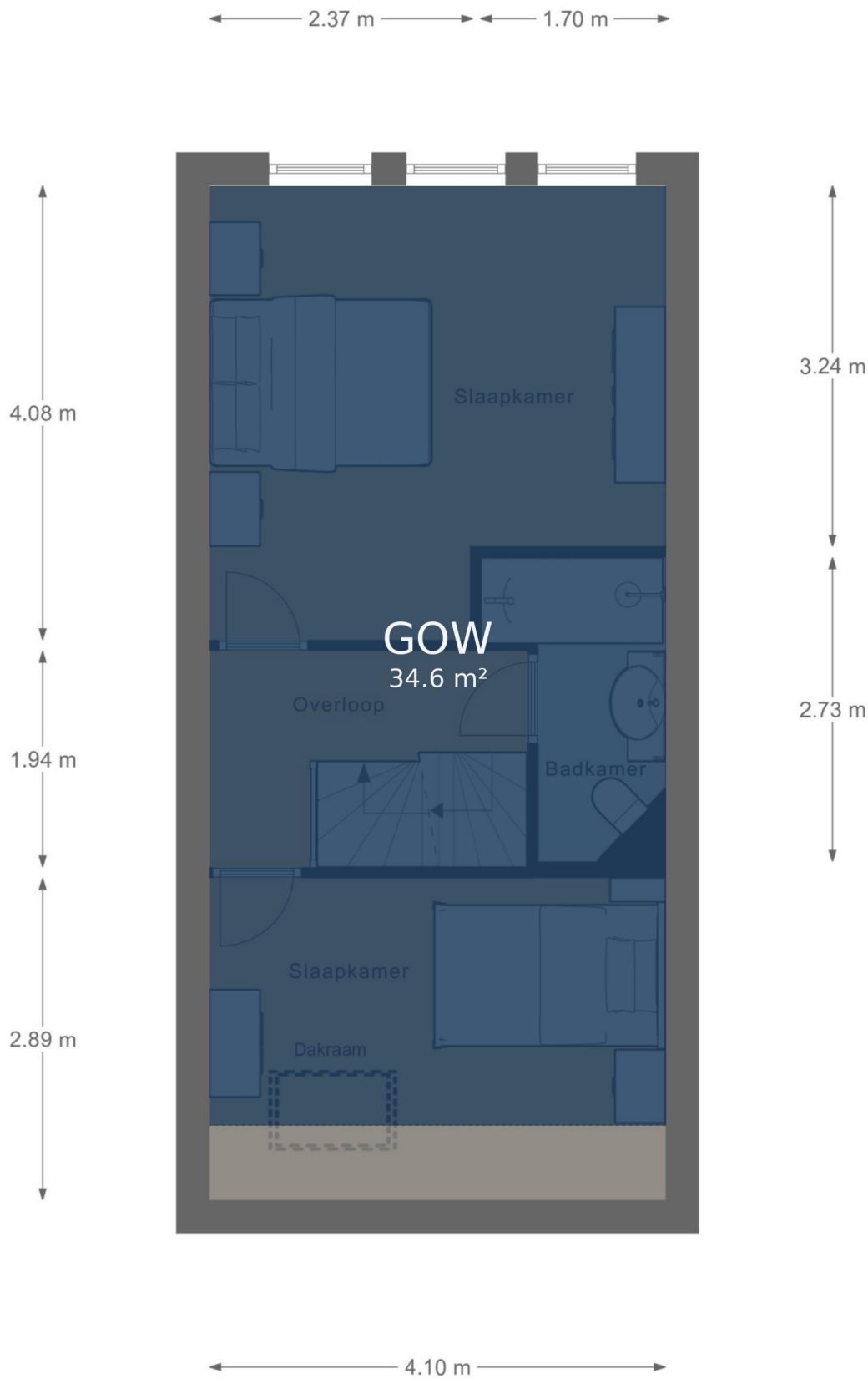
1e Verdieping
