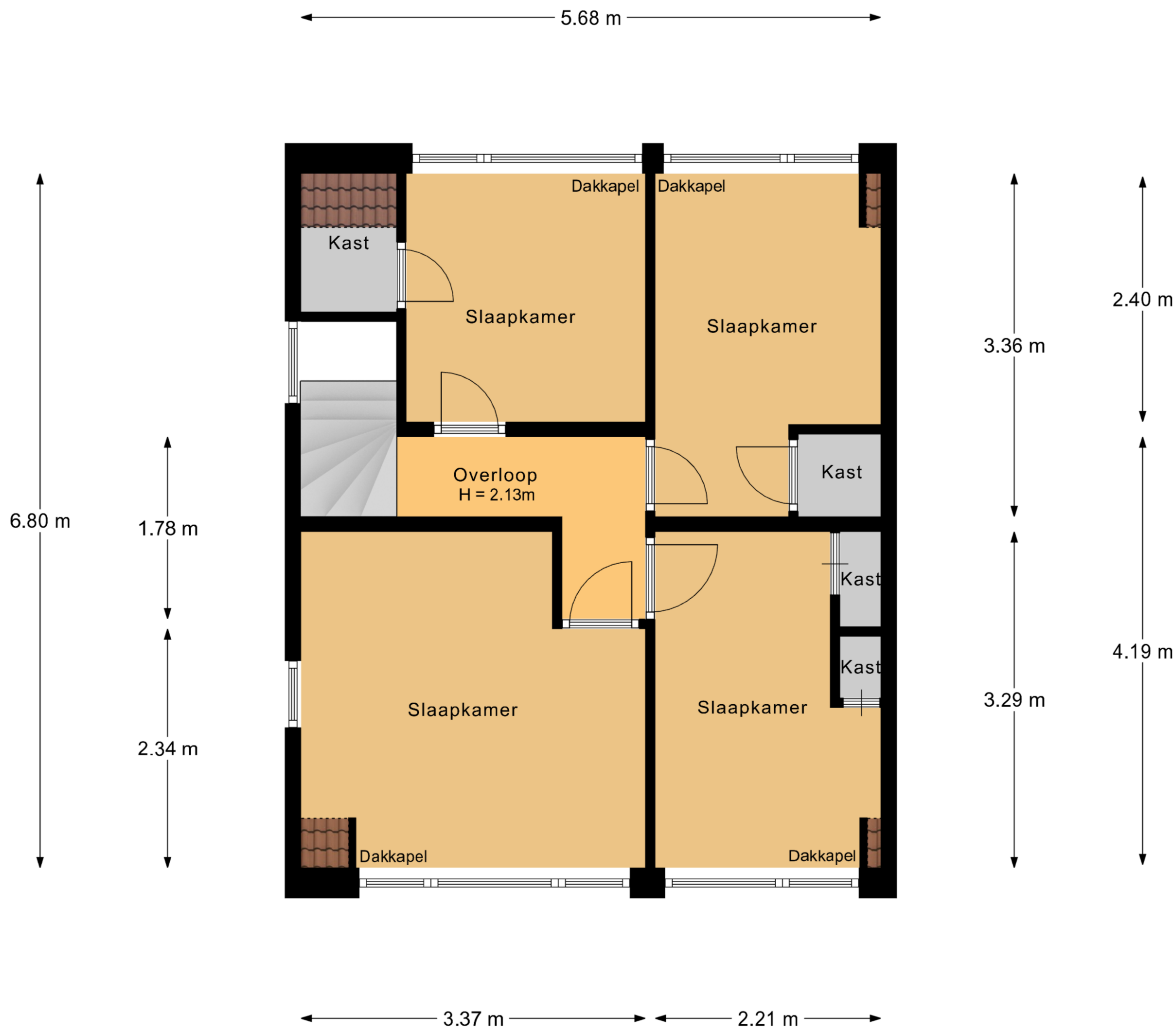
1e Verdieping
