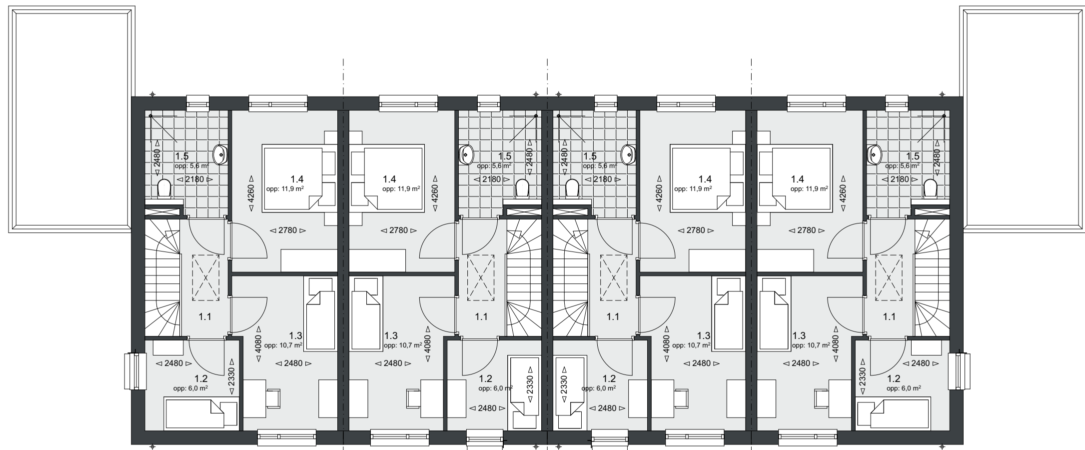
- 1e Verdieping -
