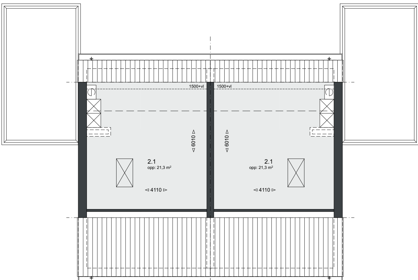
- 2e Verdieping -
