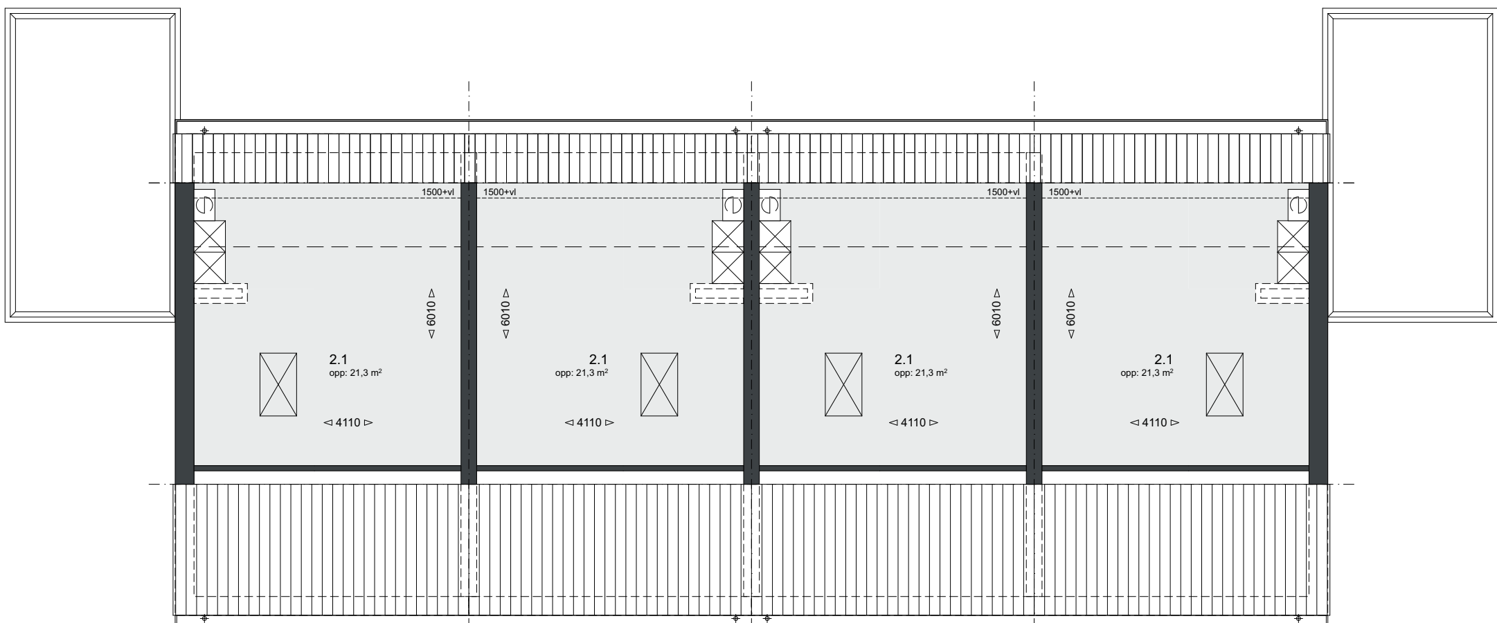
- 2e Verdieping -
