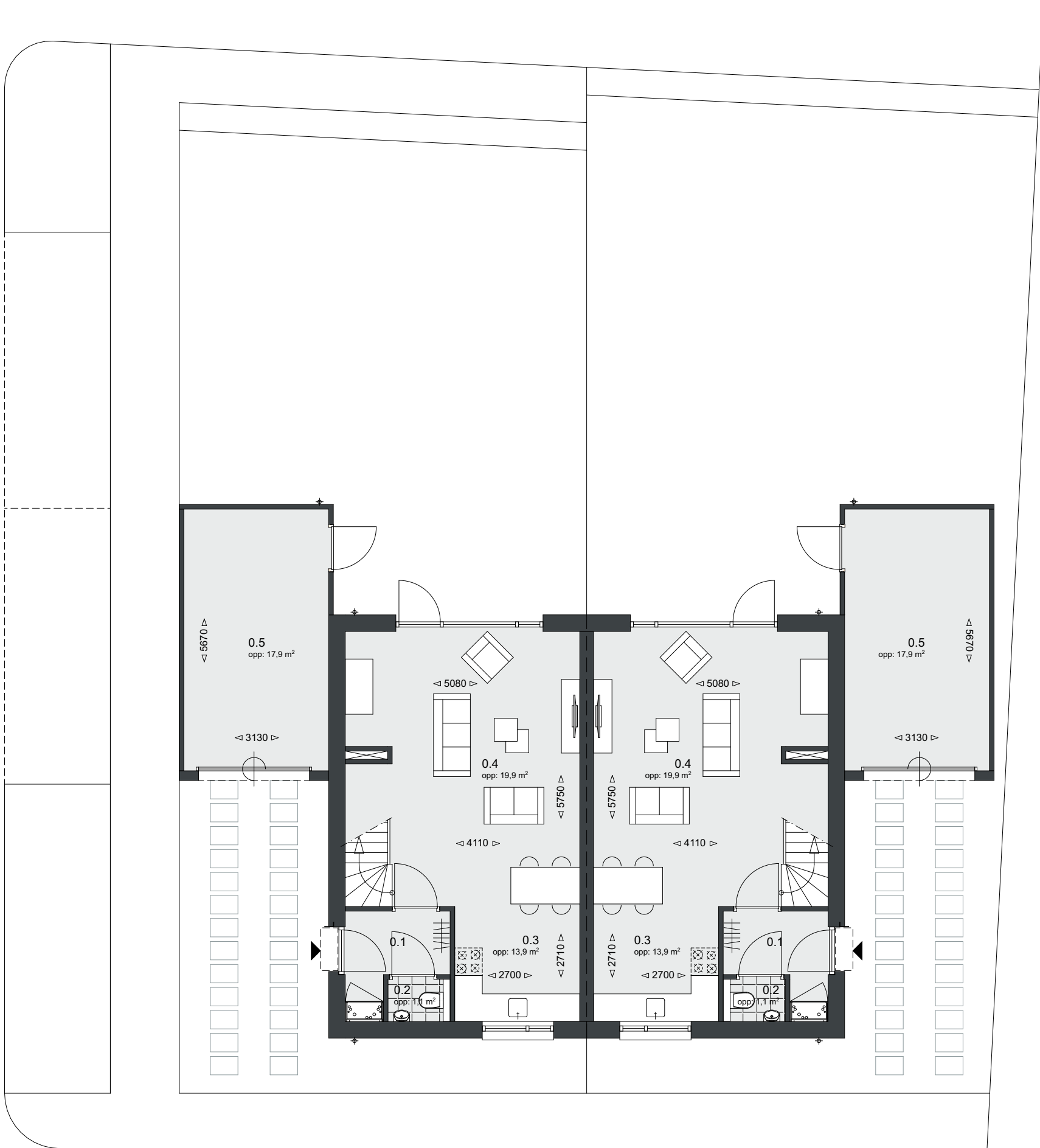
- Begane Grond -
