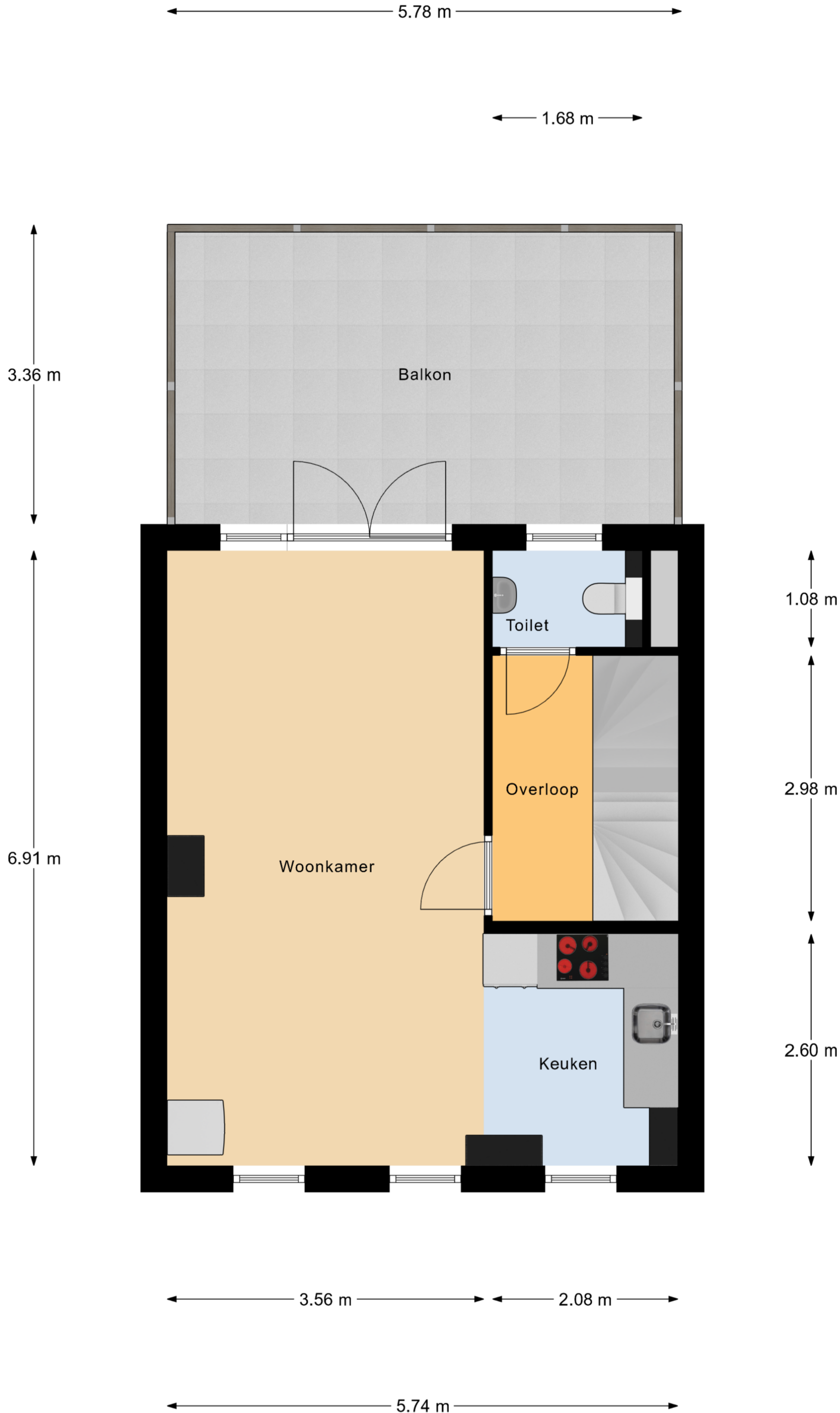
1e Verdieping
