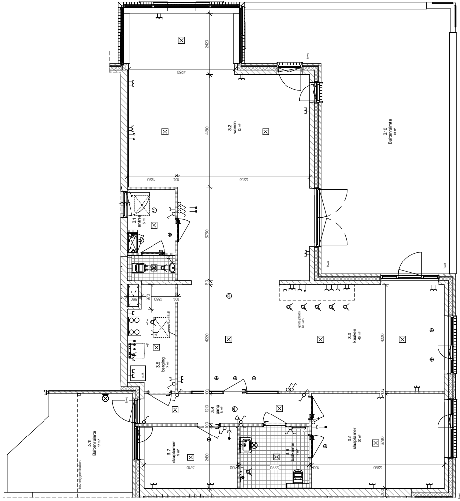
1 Begane Grond 1 : 50
